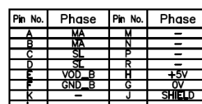
Plug : MS3102A20-29P
